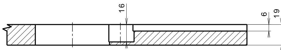
Schnittansicht A-A
