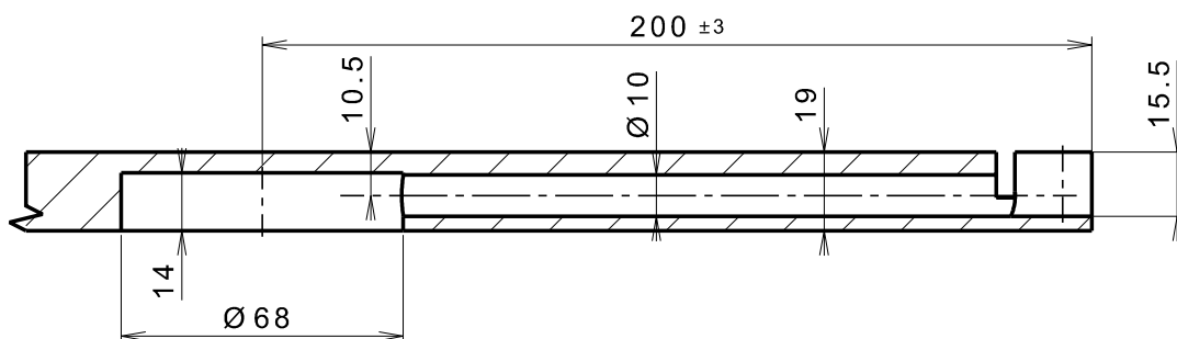
Schnittansicht A-A
