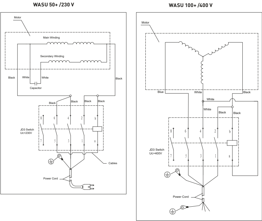
Schéma électrique
